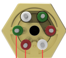
L1 L2 L3 Stjernekobling
